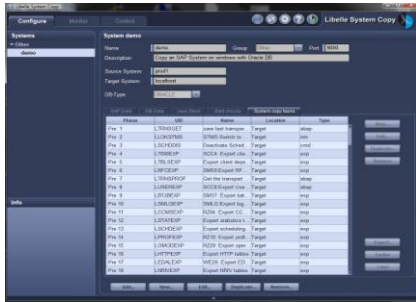
Bild Libelle_SystemCopy_Tasks_Gui.jpg:
